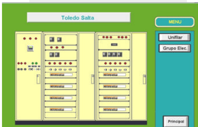
Pantalla Secundaria del software Scada de monitoreo remoto via Ethernet
